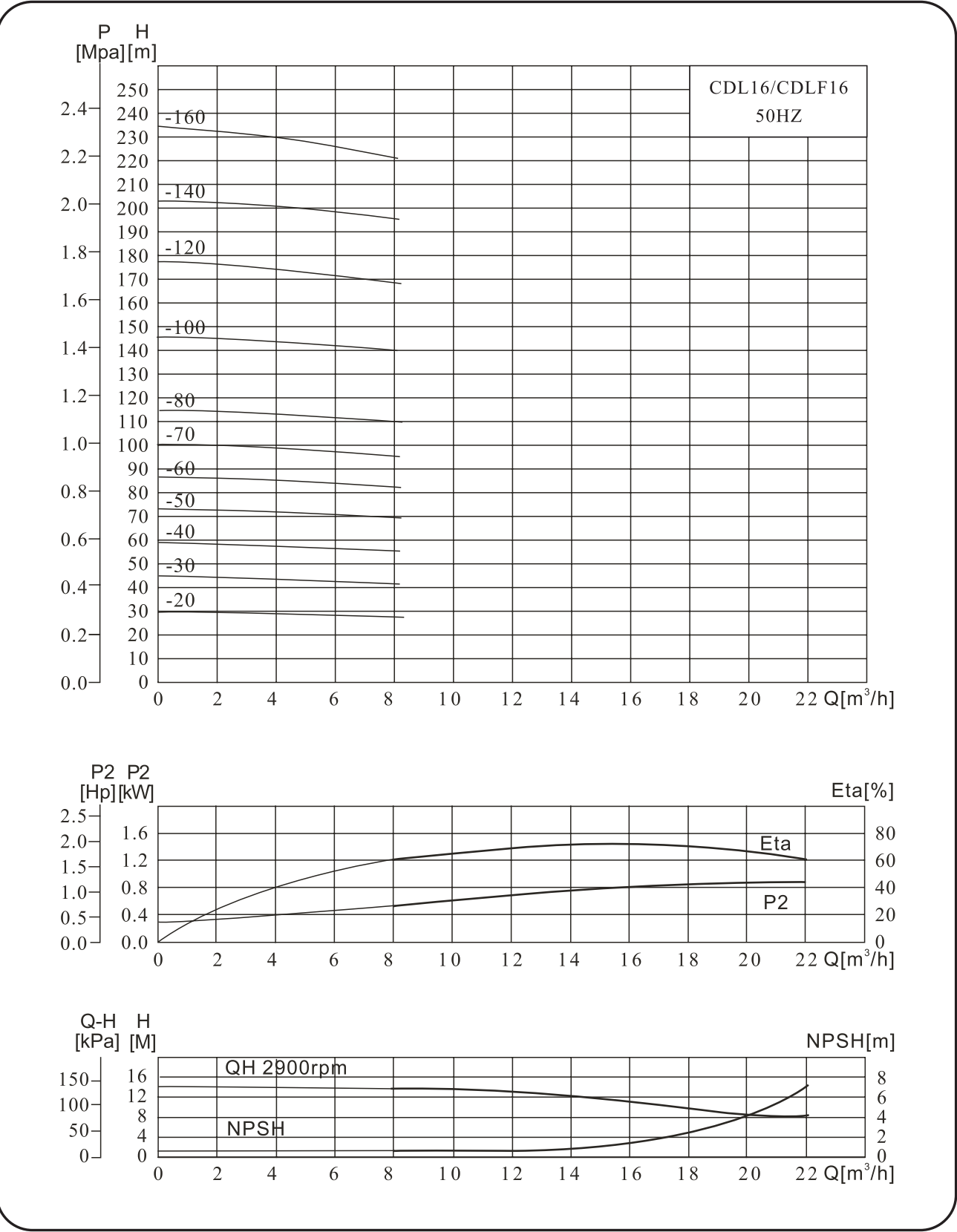
性能曲线
