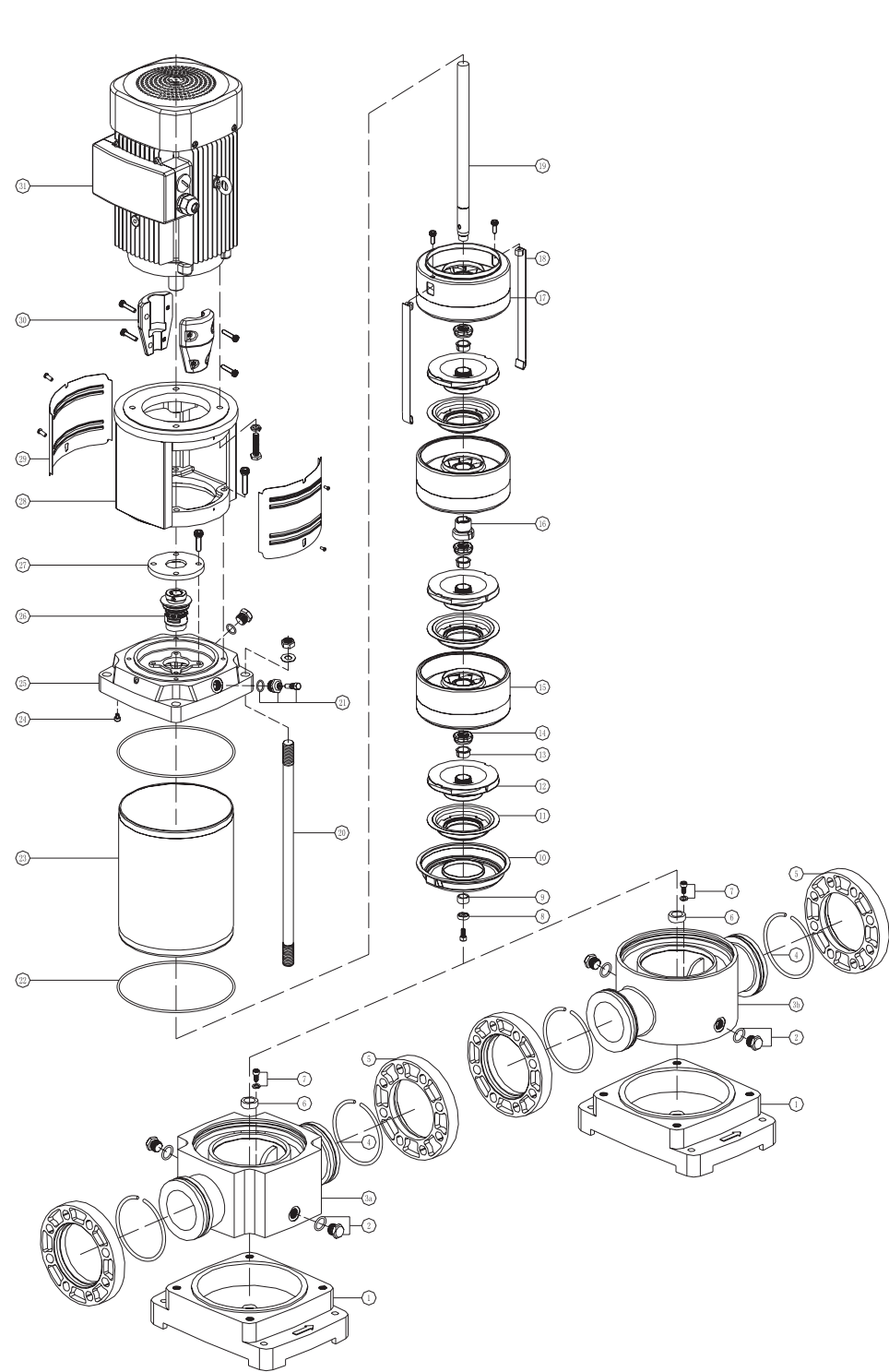
CDLF32,42,65,85 爆炸图
