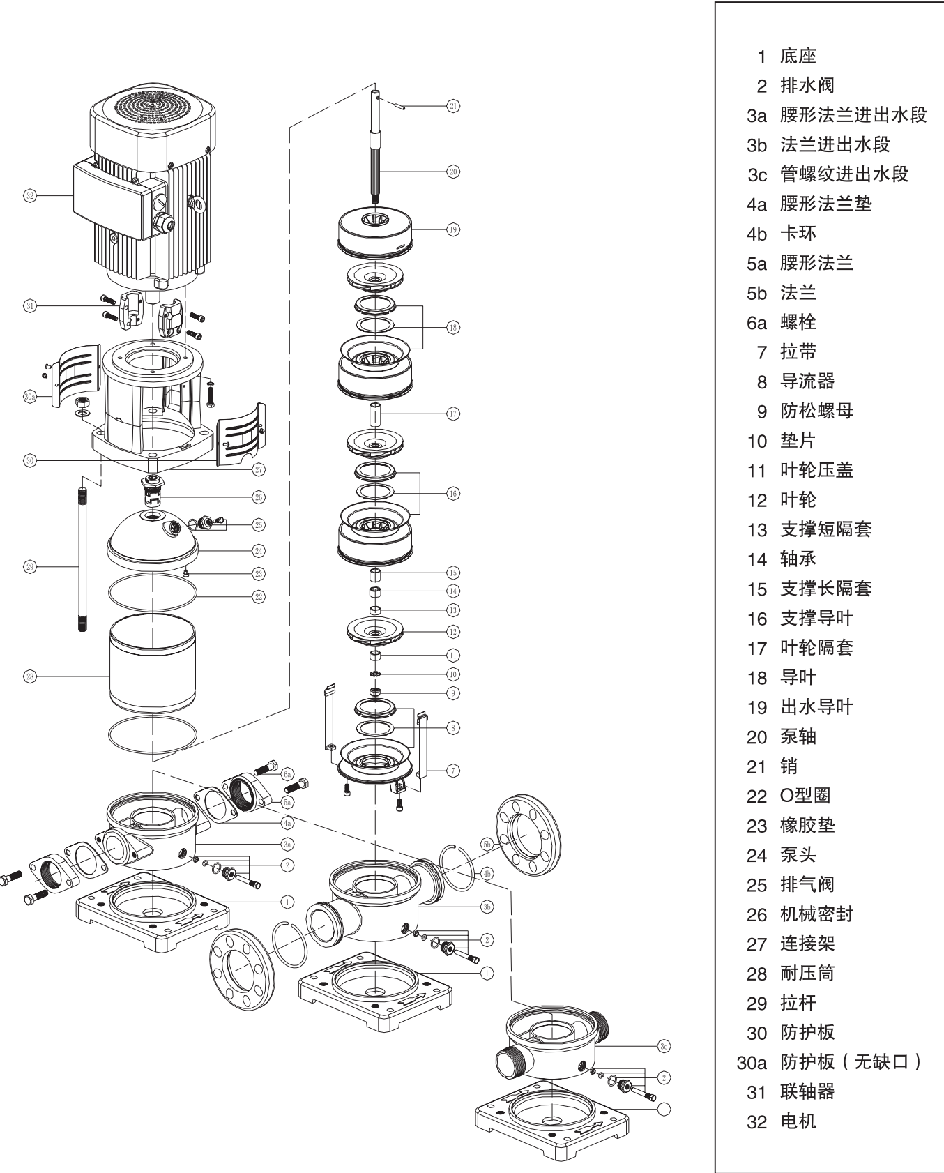
CDLF8,12,16,20 爆炸图
