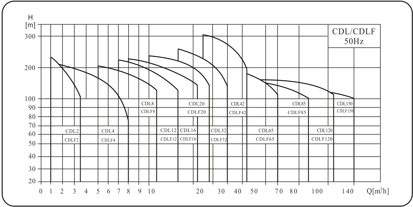
性能范围
