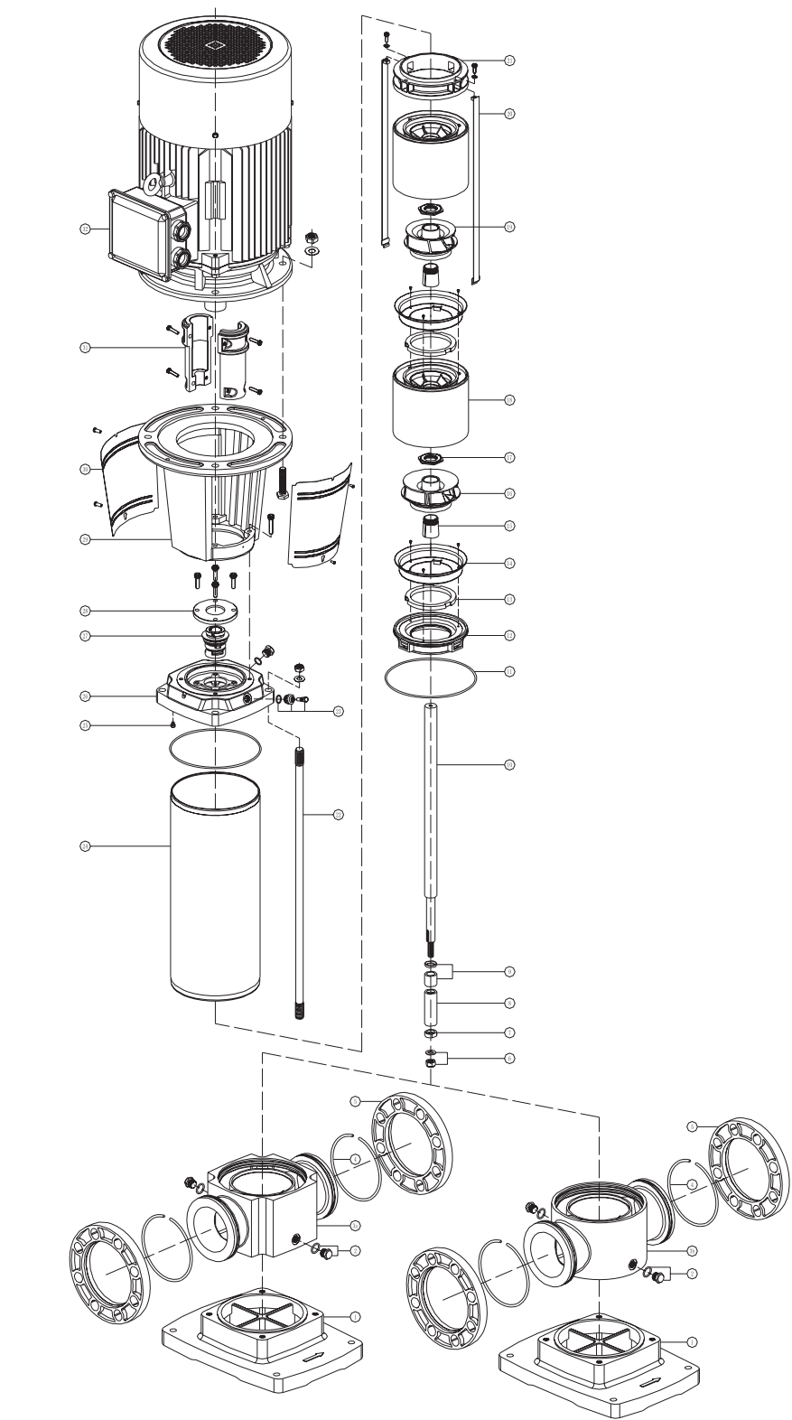
CDLF120,150 爆炸图
