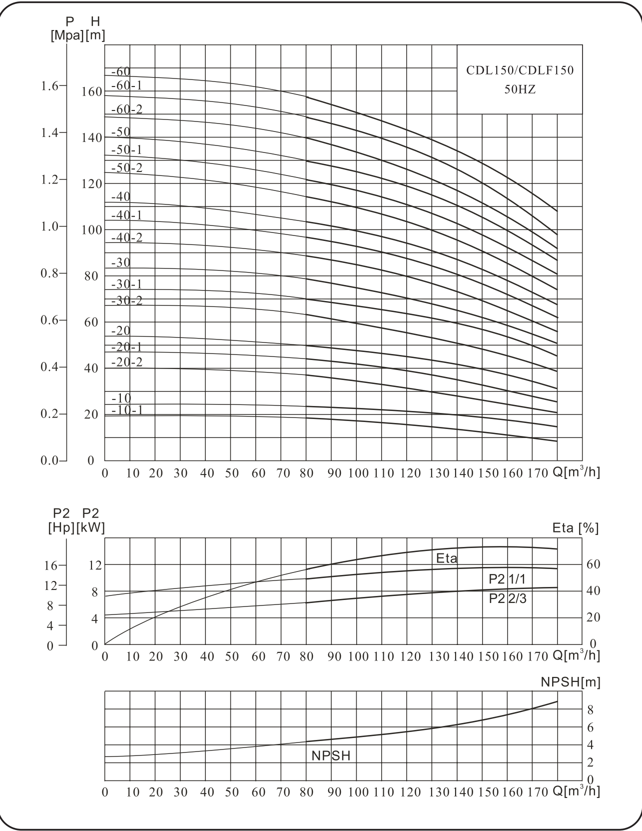
性能曲线
