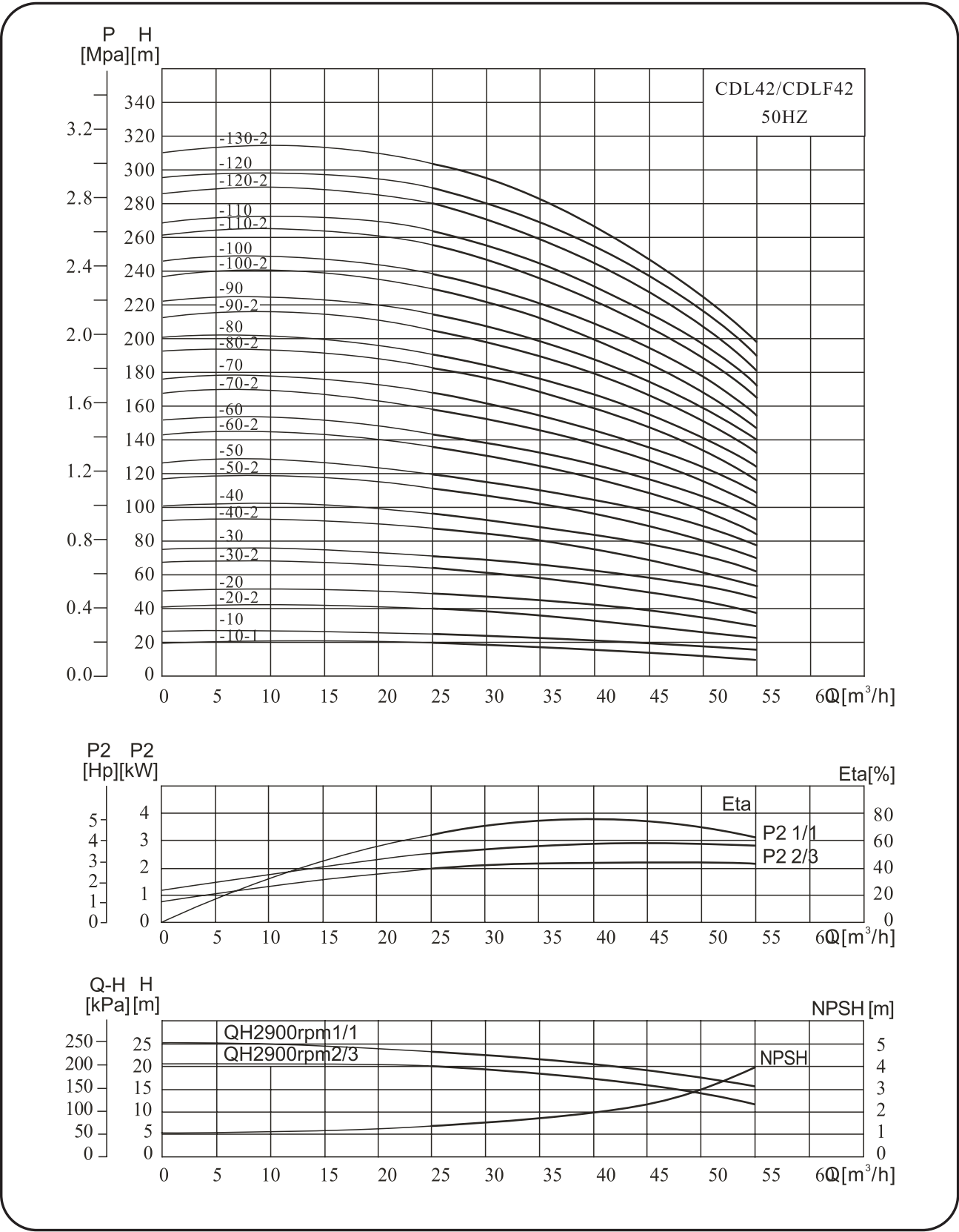
性能曲线
