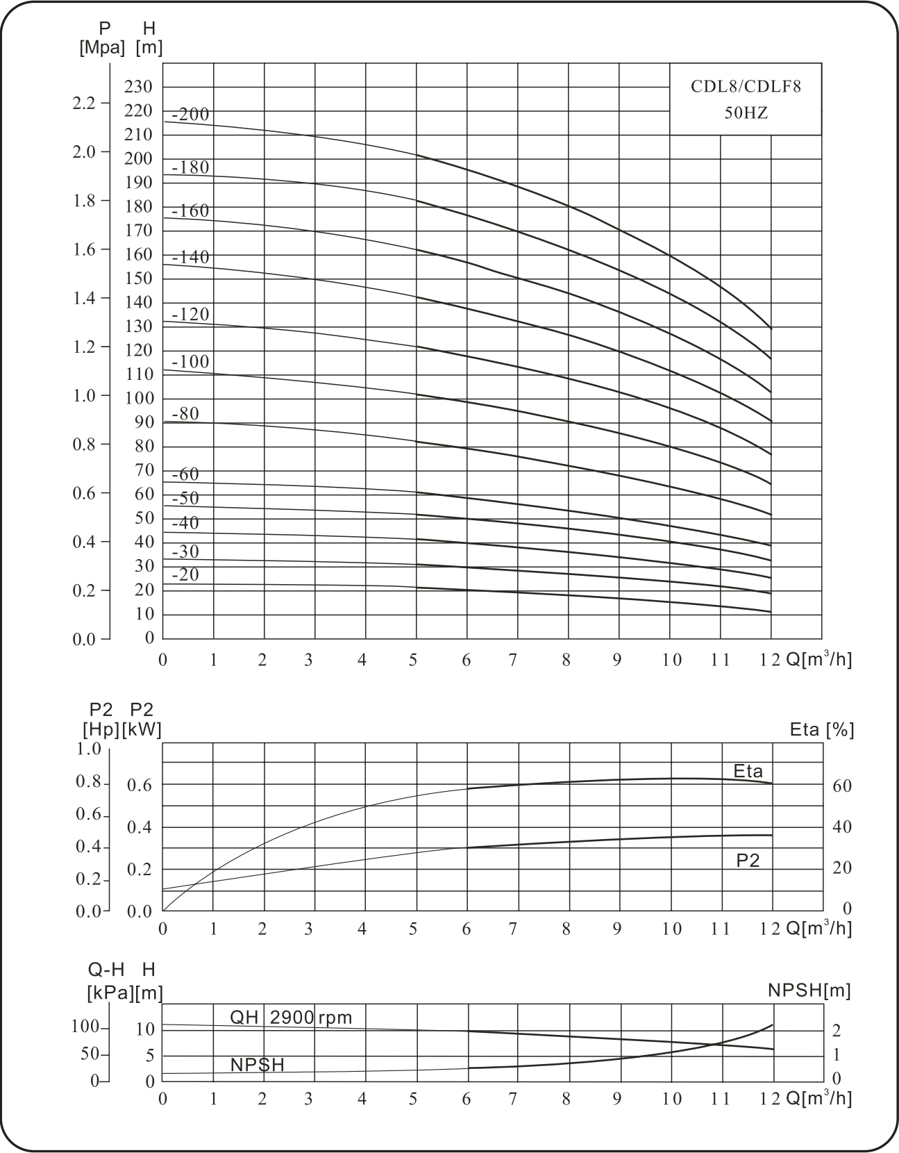
性能曲线
