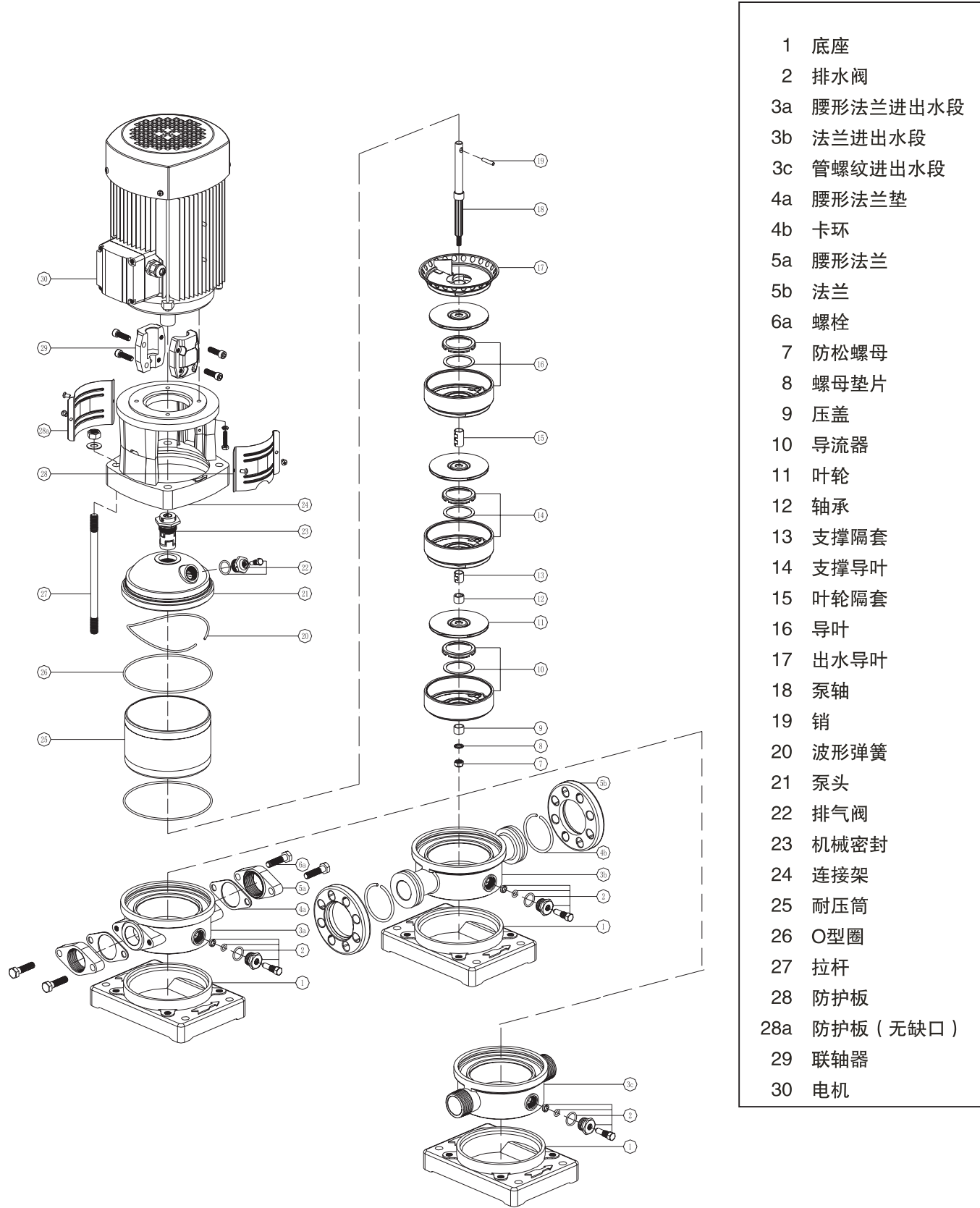
CDLF2,4 爆炸图
