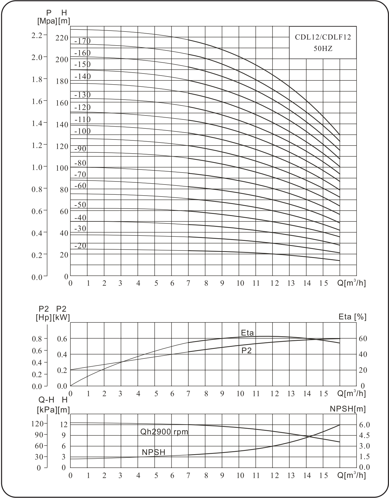
性能曲线
